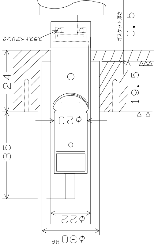
△部断面図
